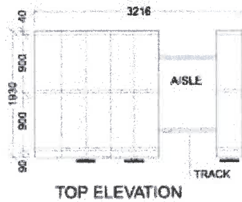
TOP ELEVATION
