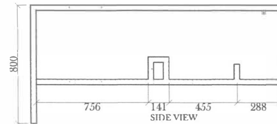
Body Frame Details Scale..... 1:25
